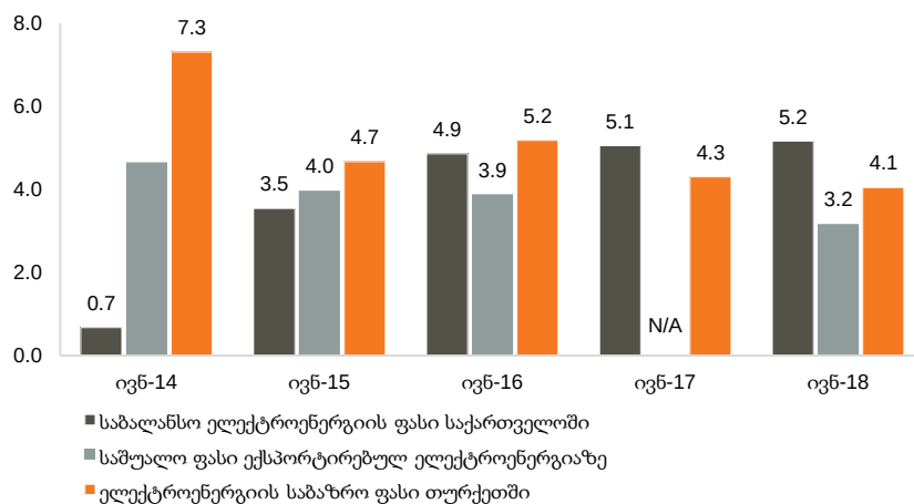
გრაფიკი 6: ელექტროენერგიის ფასები საქართველოსა და თურქეთში, აშშ ცენტი კვტ.სთ-ზე
