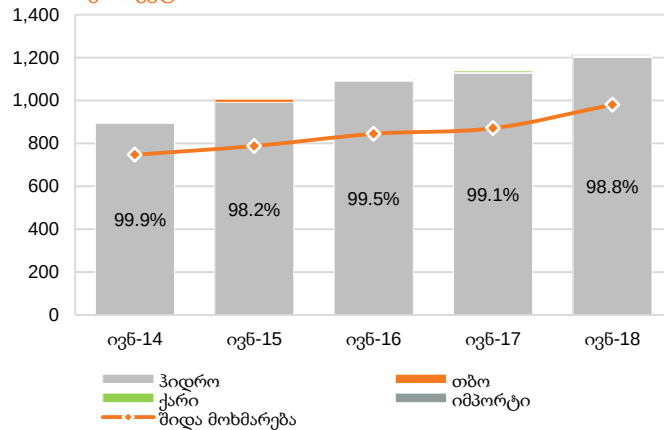
გრაფიკი 4: ელექტროენერგიის გამომუშავება, იმპორტი და მოხმარება, გვტ.სთ
